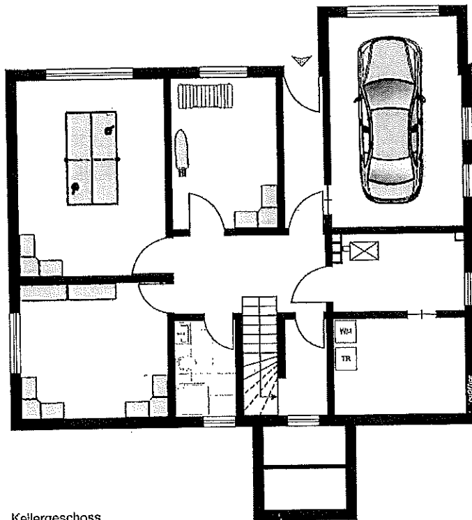
Kellergeschoss
