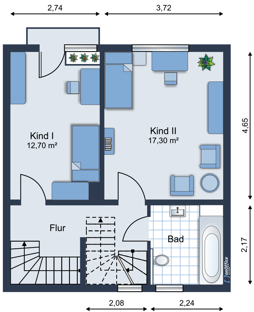
NE 3, Obergeschoss
